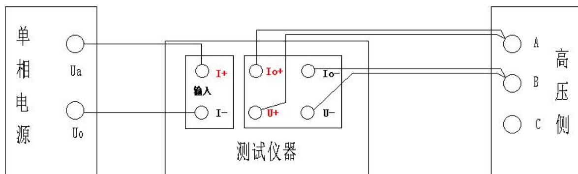
图8 星接-单相直接接线图
