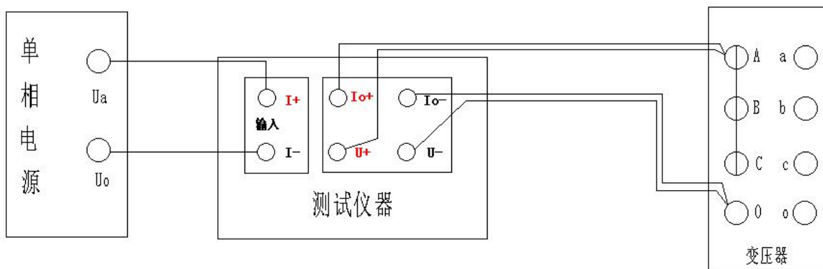
图 15 零序阻抗直接接线图
