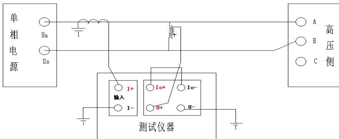
图9 星接-单相外接电压互感器和电流互感器接线图
