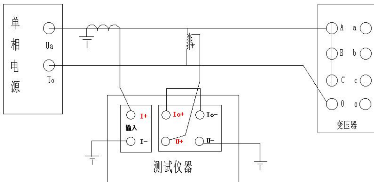
图 16 零序阻抗外接电压互感器、外接电流互感器接线图
