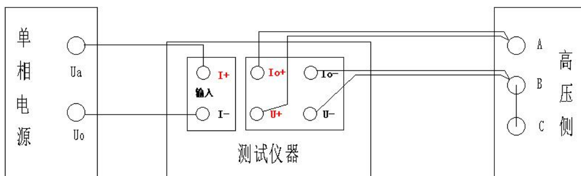
图 10 △接-直接接线图
